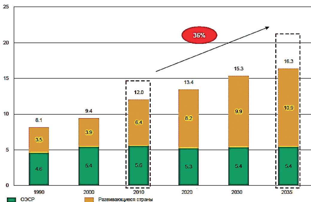
Рис. 1. Мировое потребление энергоресурсов в 1990—2035 гг., млрд т н.э. [9]
